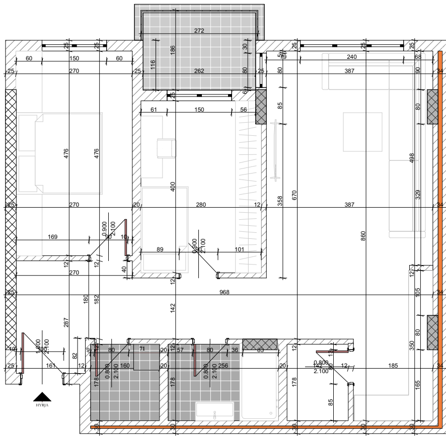
Tipi F LLAMELLA R2 91.70m 2 Kati-II,III,IV,V,VI
