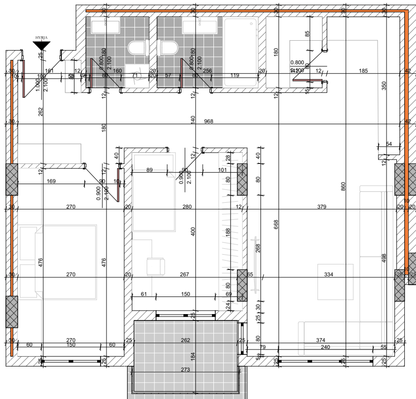
Tipi C LLAMELLA R2 90.76m 2 Kati-II,III,IV,V,VI
